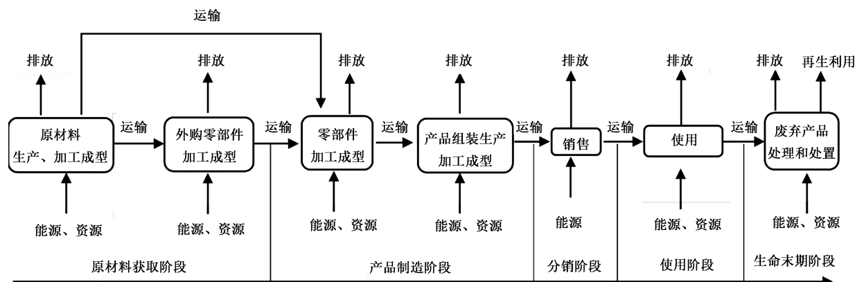
图1 房间空调器产品碳足迹量化的系统边界示例
