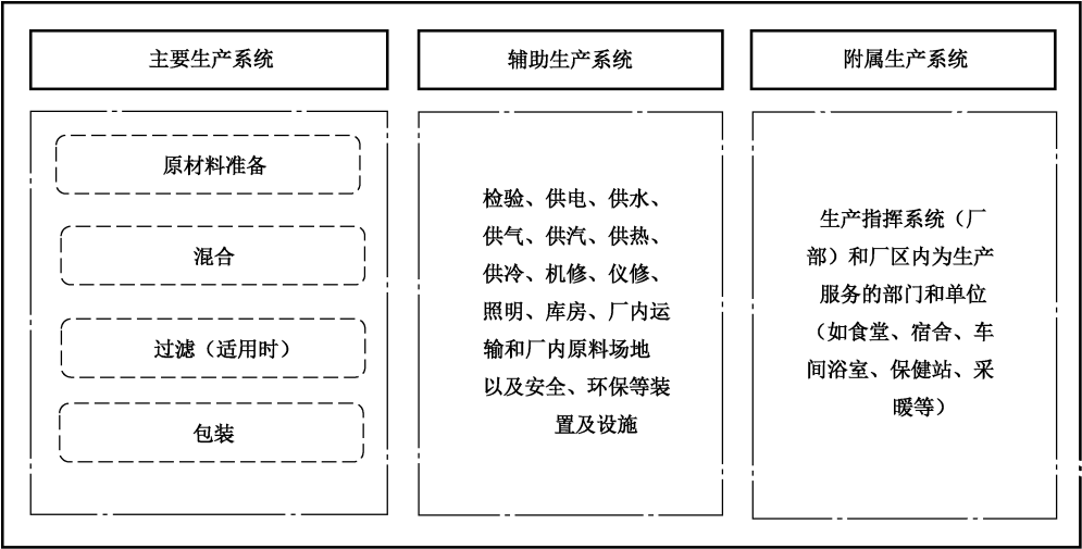
图 A.3 水泥基防水材料生产企业温室气体排放核算边界示意图
