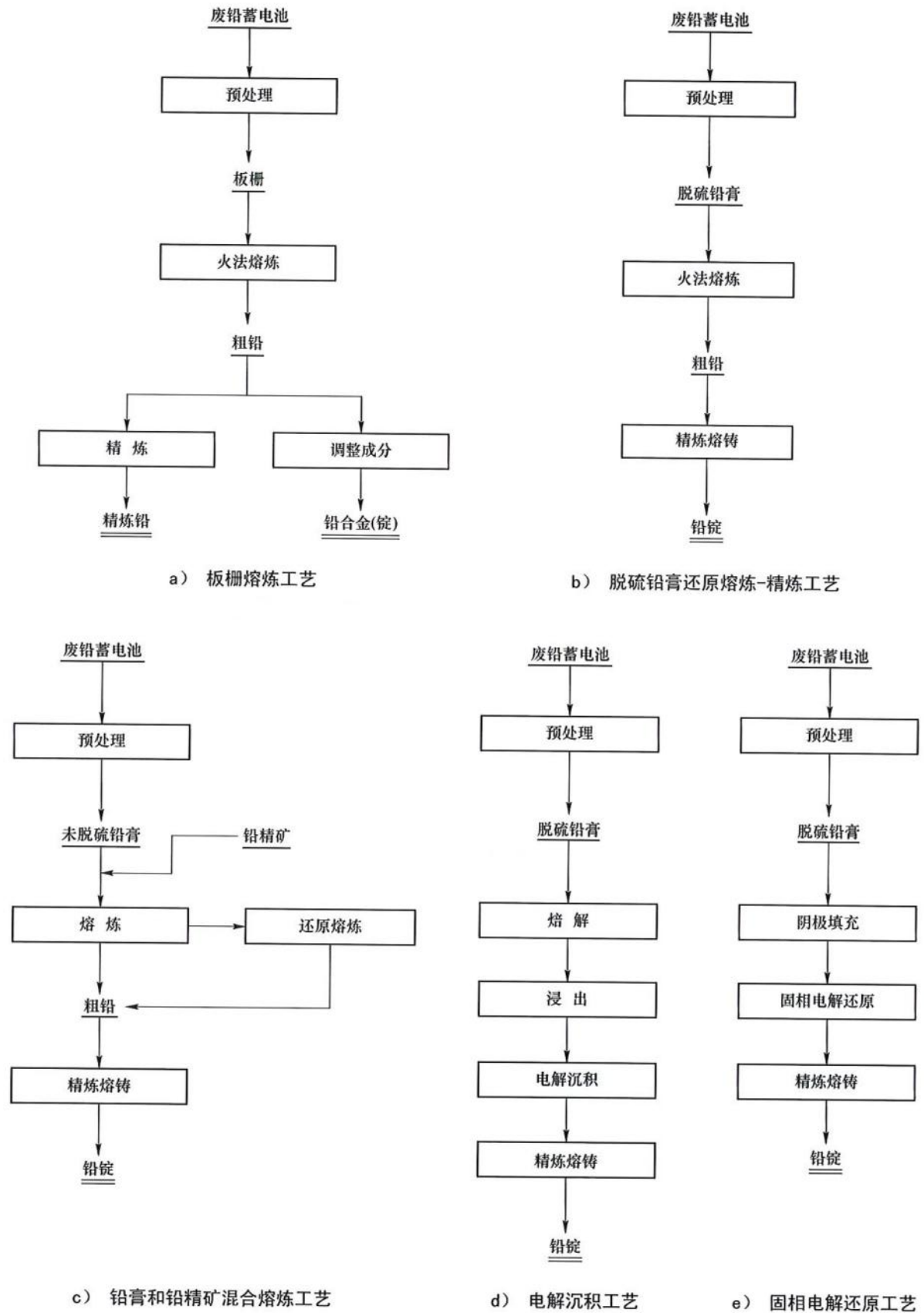
图 A.2 以废铅蓄电池拆解后含铅废料为原料的主要工艺路线
